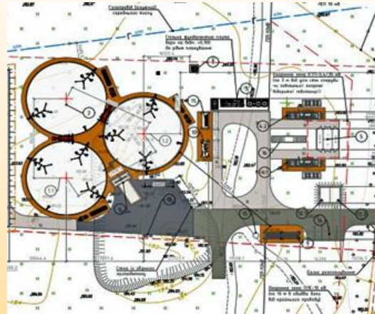
Біогазовий комплекс 1,5 МВт с.Чорний Ріг, Чернігівська область
